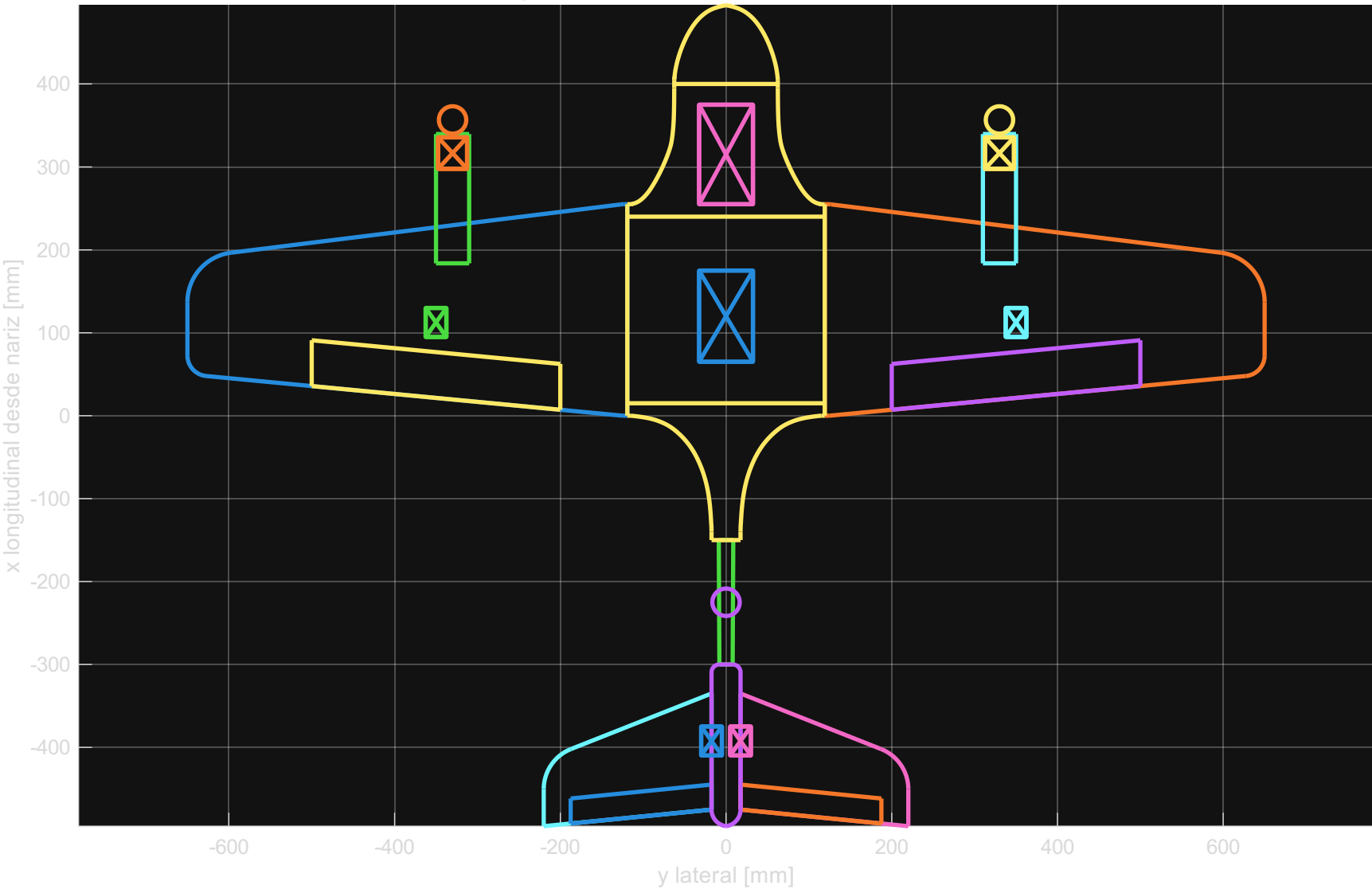
Partes DXF separadas - sin reconstrucción artificial de contornos
